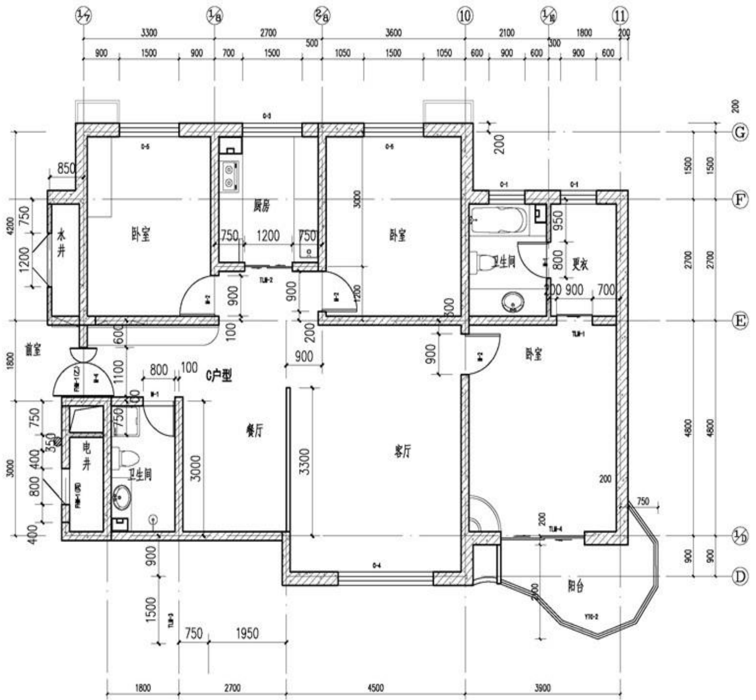
16#楼C户型平面图 150
