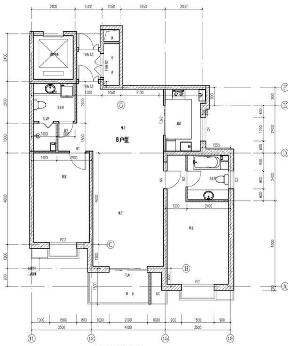
17#楼B户型(东侧)平面图 150
