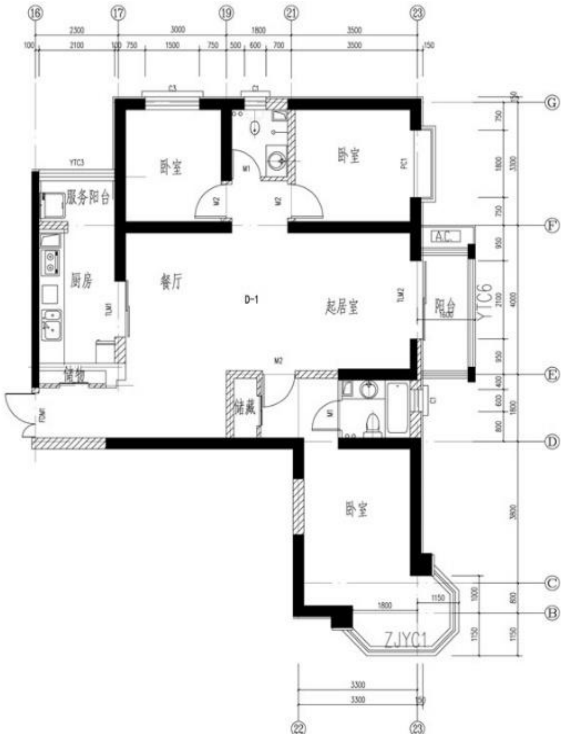
10#、13#楼D-1户型平面图 1:50
