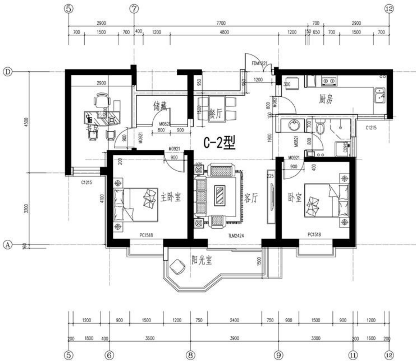
17#、21#楼C-2户型平面图 1:50
