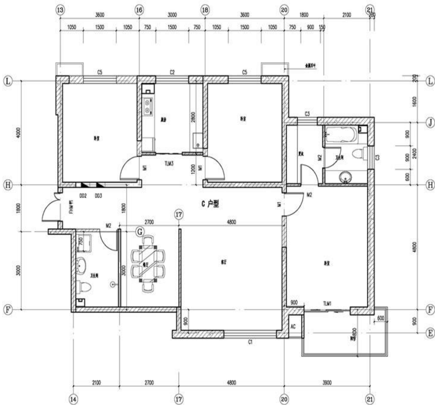
17#楼C户型平面图 150
