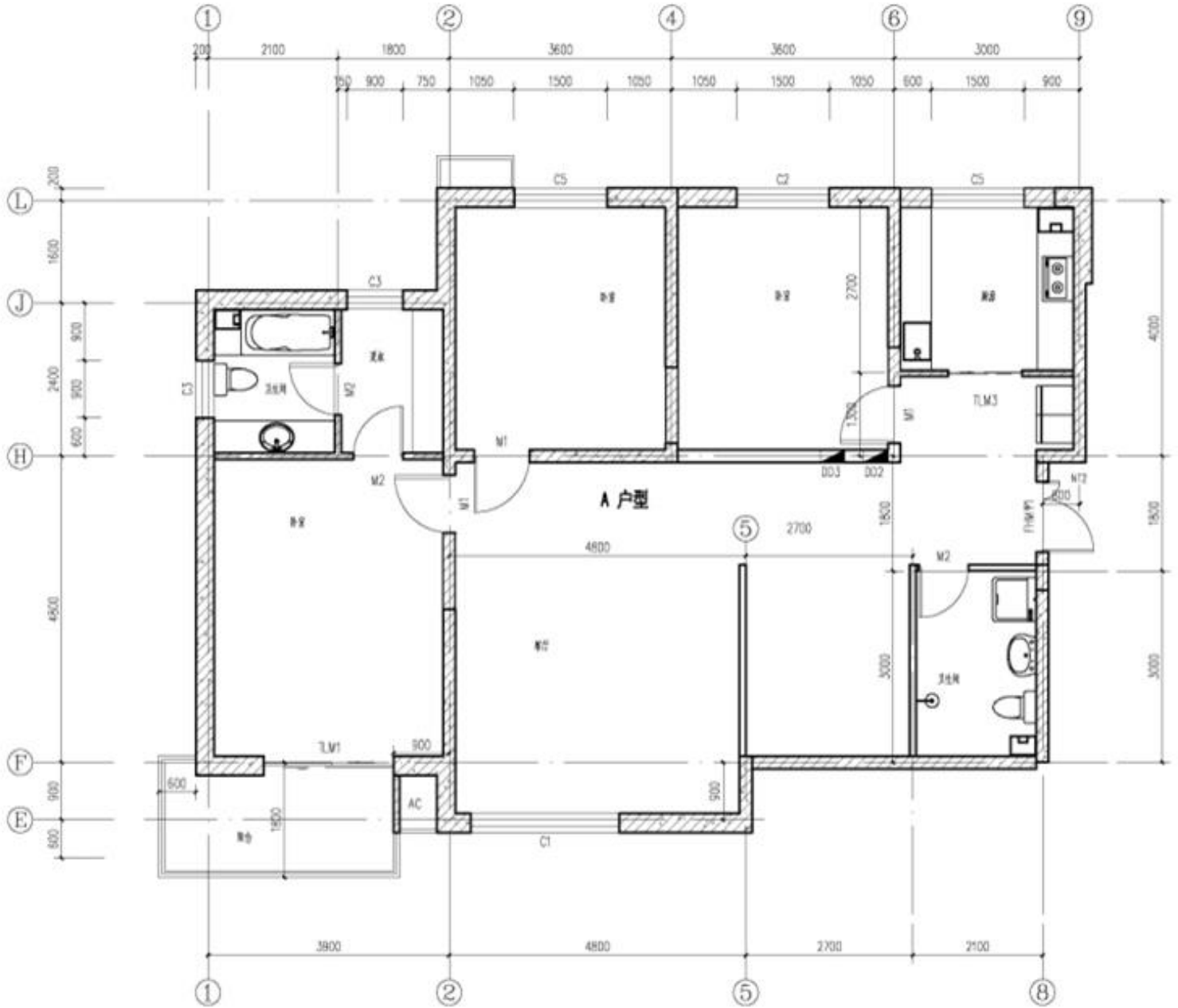
17#楼A户型平面图 150
